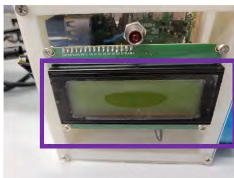
顯示屏：小童走進廚房時會即時顯示文字，讓傭工或家人得知小童走進廚房。
